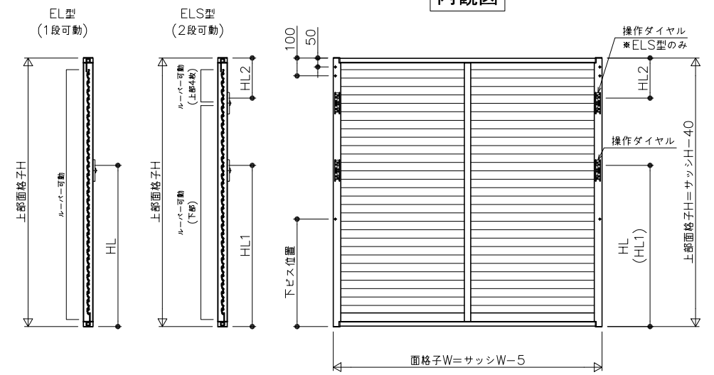
内観図
